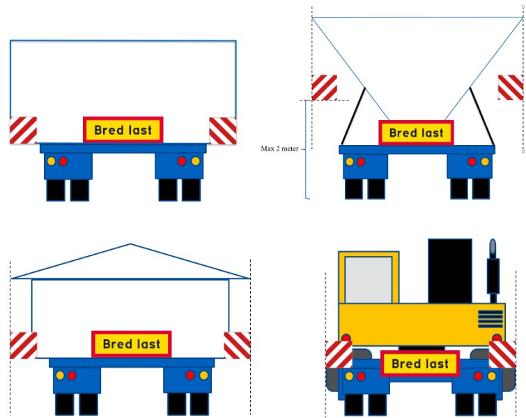
Figura 1. Poziția semnelor de marcare a lățimii în direcția orizontală.
