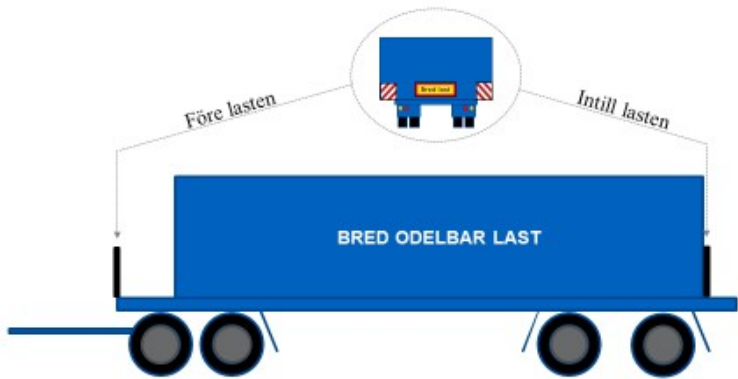
Figura 2. Poziția semnelor de marcare a lățimii în direcția longitudinală pe încărcătură.
