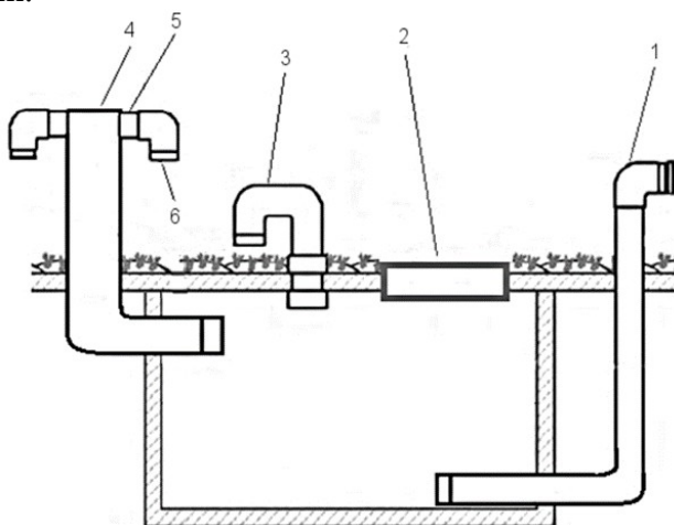
Rys. 1. Przykład zbiornika na wodę: 1 – sucha rura ze złączką B(75) o rozmiarze PN16 [9.10]; 2 – zamykana pokrywa inspekcyjna; 3 – otwór wentylacyjny; 4 – rura o średnicy 100 mm; 5 – zawór zwrotny; 6 – złączka B(75) o rozmiarze PN16 [9.10] do uzupełniania wody.
