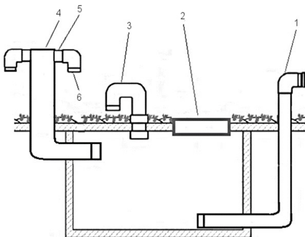
Figura 1. Exemplo de um tanque de água: 1 — tubo seco com manga de acoplamento tamanho B(75) de tamanho PN16 [7.10]; 2 — capa de inspeção bloqueável; 3 — orifício de ventilação; 4 — tubo com um diâmetro de 100 mm; 5 — válvula antirretorno; 6 — Manga de acoplamento de tamanho B(75) PN16 [7.10] para reabastecimento de água.
