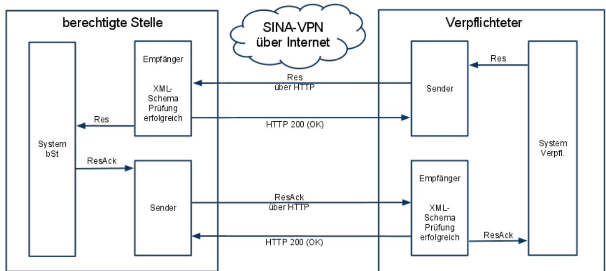
Abbildung 6: erfolgreiche Übermittlung einer Response
