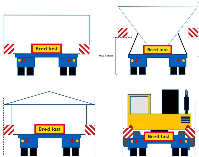
Slika 1. Položaj znakov za označevanje širine v vodoravni smeri.
