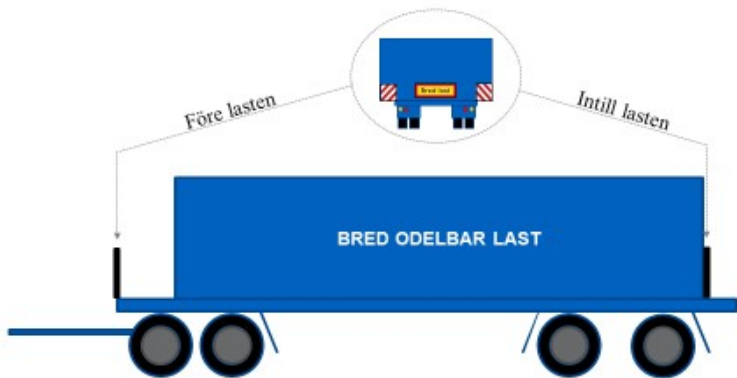
Slika 2. Položaj oznak za označevanje širine v vzdolžni smeri tovara.
