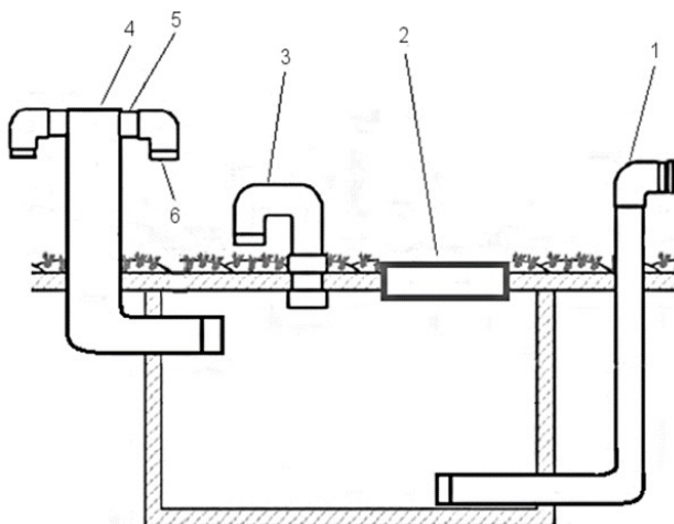
Figure 1. Exemple de réservoir d'eau: 1 — tuyau sec avec manchon d'attelage PN16 de taille B(75) [7.10]; 2 — couverture d'inspection verrouillable; 3 — orifice de ventilation; 4 — tube d'un diamètre de 100 mm; 5 — soupape de non-retour; 6 — manchon d'attelage PN16 de taille B(75) [7.10] pour le réapprovisionnement en eau.
