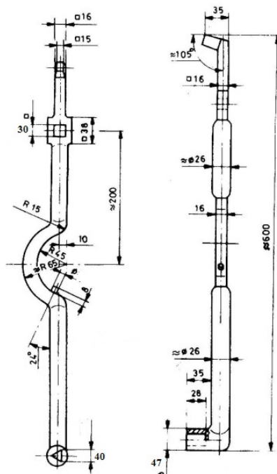
Figure 2. Clé de bouche d'incendie au sol
