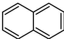
Naphtil–
