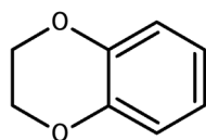
Etilendioksifenil-Furil–
