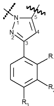
Pirazol-1,5-diilas
