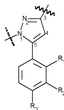
Pirazol-1,3-diilas
