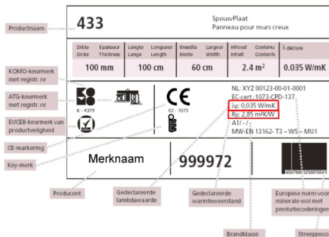
Figuur 47: CE markering op een isolatieplaat
