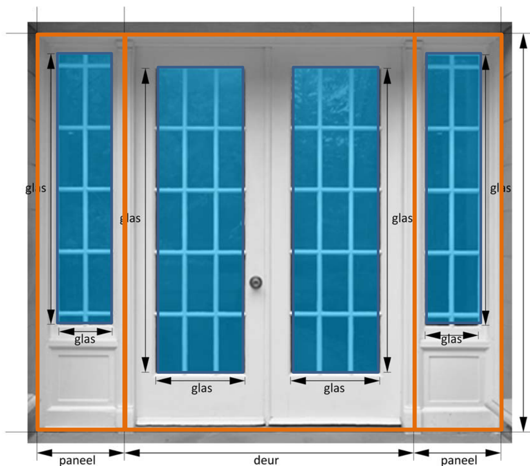
Figuur 45: Voorbeeld van een opening bestaande uit zowel deur (met glas) als paneel (met glas). De panelen (de vaste delen links en rechts zonder de beglazing), de deuren (de opengaande opake delen in het midden zonder de beglazing) en de beglazingen worden elk apart ingevoerd in de software. Het glas is hier niet vastgezet met aparte profielen en is ingewerkt in de dikte van het hout à type profiel 'geen'.
