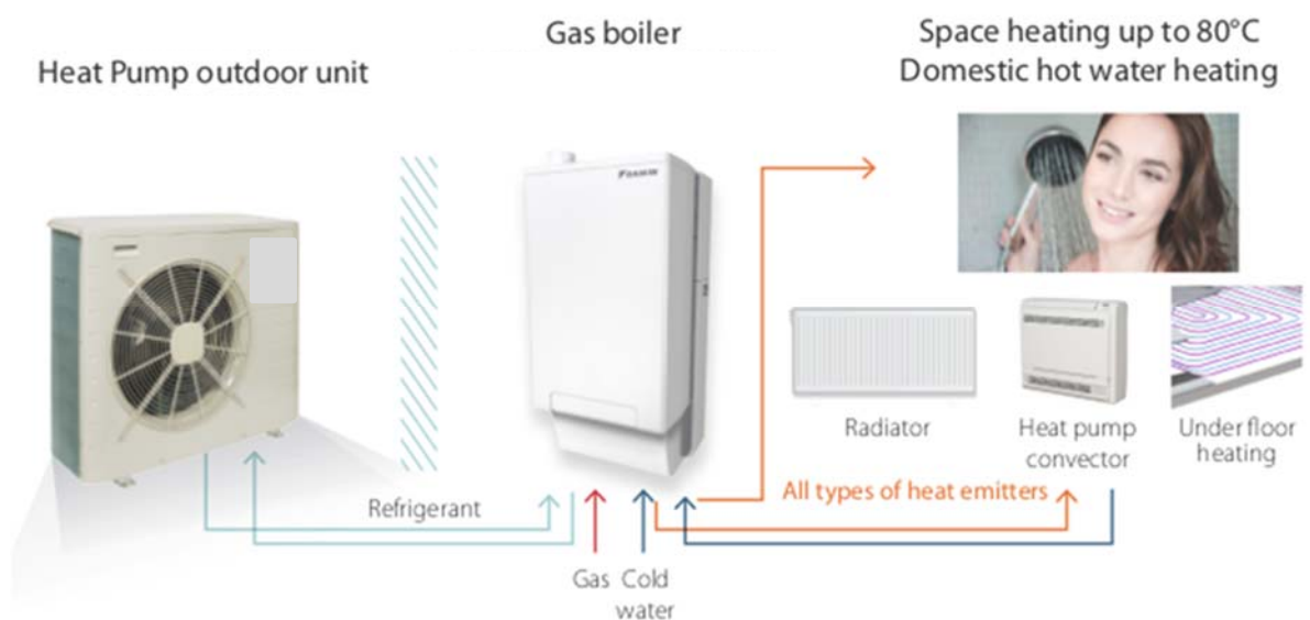
Figuur 147: Werking van een hybride warmtepomp
