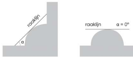
Figuur 42: Voorbeeld: bepalen van de helling van een lichtstraat en koepel in een plat dak
