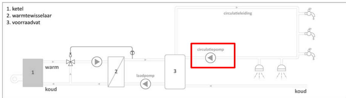
Figuur 218: Circulatieleiding met circulatiepomp bij een voorraadvat
