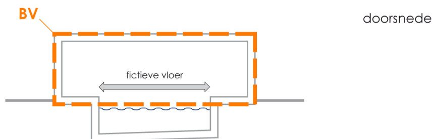
Figuur 19: Zwembad: vereenvoudiging en fictieve vloer
