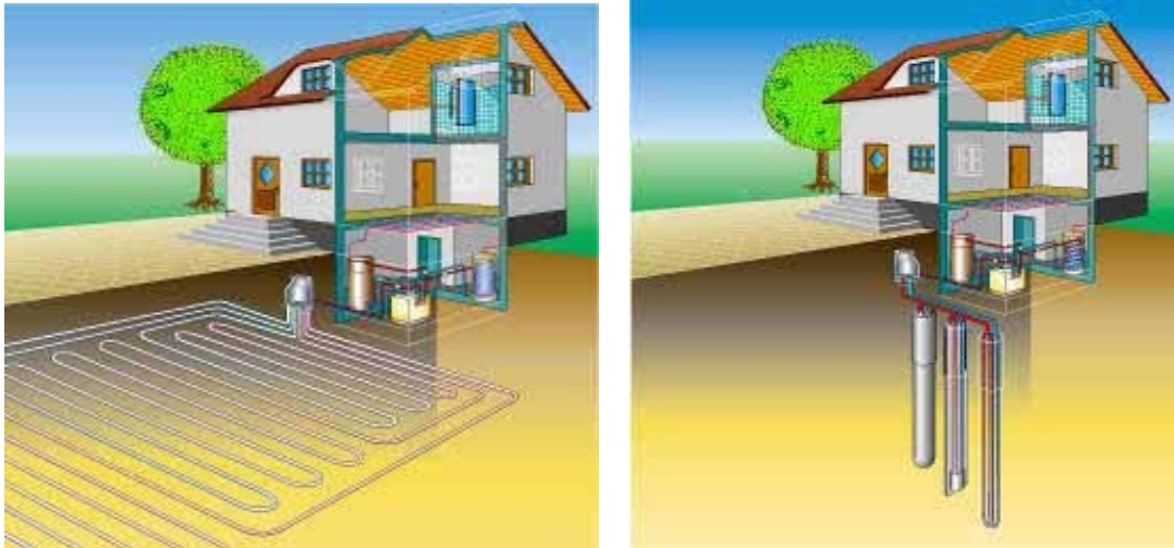
Figuur 193: Schematische voorstelling van een bodem/water koude-opwekker met horizontale bodemwarmtewisselaar (links) en met verticale bodemwarmtewisselaar gesloten systeem (rechts)
