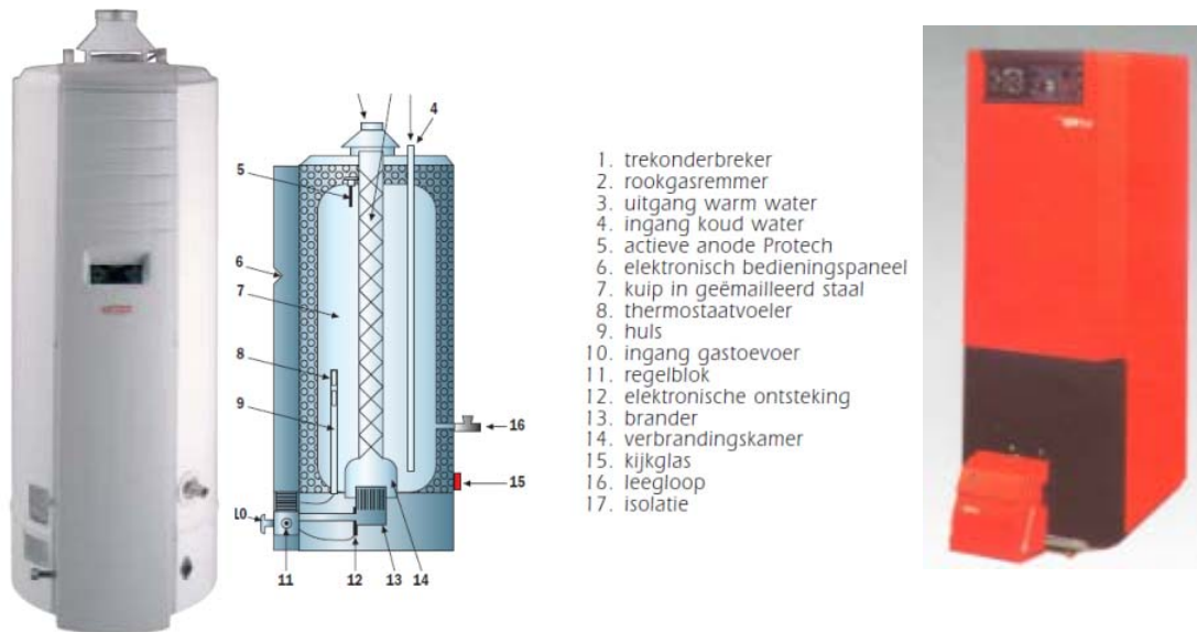
Figuur 215: Voorraadvat met geïntegreerde gasbrander (links) en met geïntegreerde stookoliebrander (rechts)
