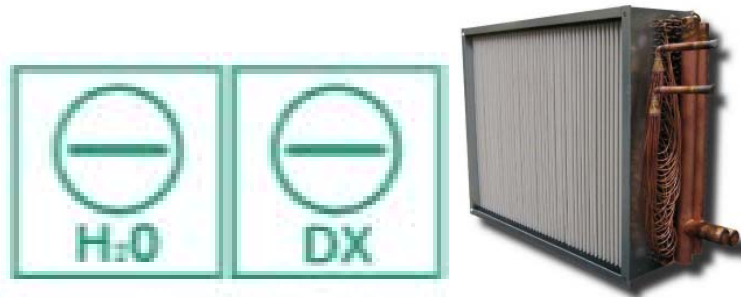
Figuur 196: Voorbeelden van symbolen voor koelbatterijen in luchtbehandelingskasten ijswater (links) en directe verdamping (midden), koelbatterij (rechts)
