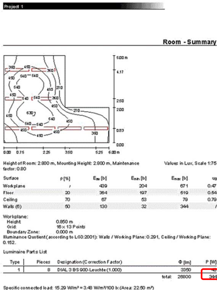
Figuur 245: Voorbeeld van verlichtingsstudie uitgevoerd met gespecialiseerde software
