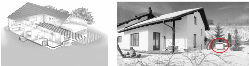
Figuur 143: Werkingsprincipe en foto buitenunit buitenlucht/water systeem
