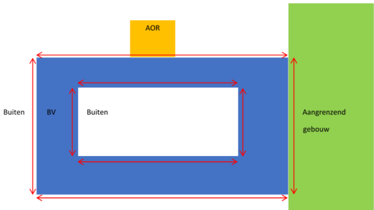
Figuur 65: Voorbeeld van de inschatting van de lengte van een circulatieleiding of combilus
