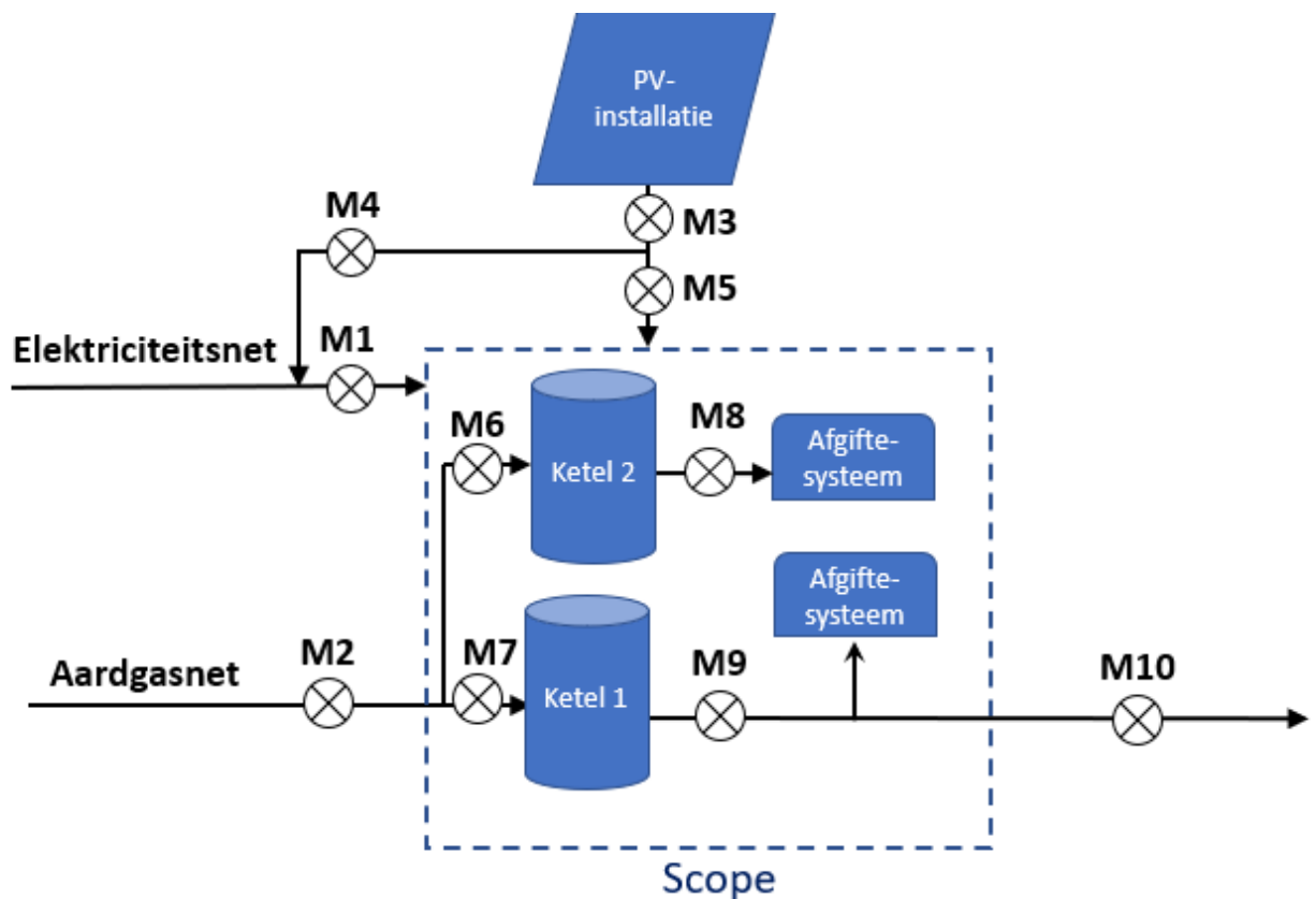
Figuur 2: voorbeeld verplichte en optionele metingen
