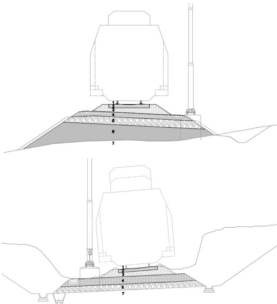
Slika 2.3: Shematski prikaz ceste v nasipu in vkopu: 1 – krovna plast, 2 – stabilizirana nosilna plast, 3 – ZNNP (nevezana nosilna plast), 4 – SNNP (kamnita posteljica), 5 – zaključna plast nasipa, 6 – nasip, 7 – temeljna tla
