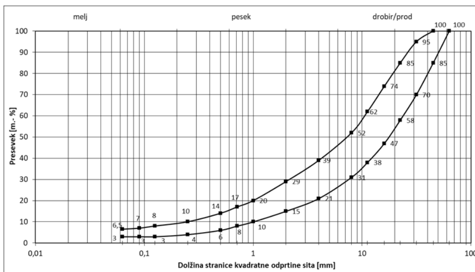
Slika 3.4: Območje sestave agregata 0/45 mm za ZNNP in NOP za vgradnjo
