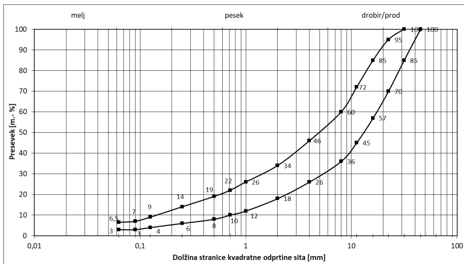
Slika 3.3: Območje sestave agregata 0/32 mm za ZNNP in NOP za vgradnjo
