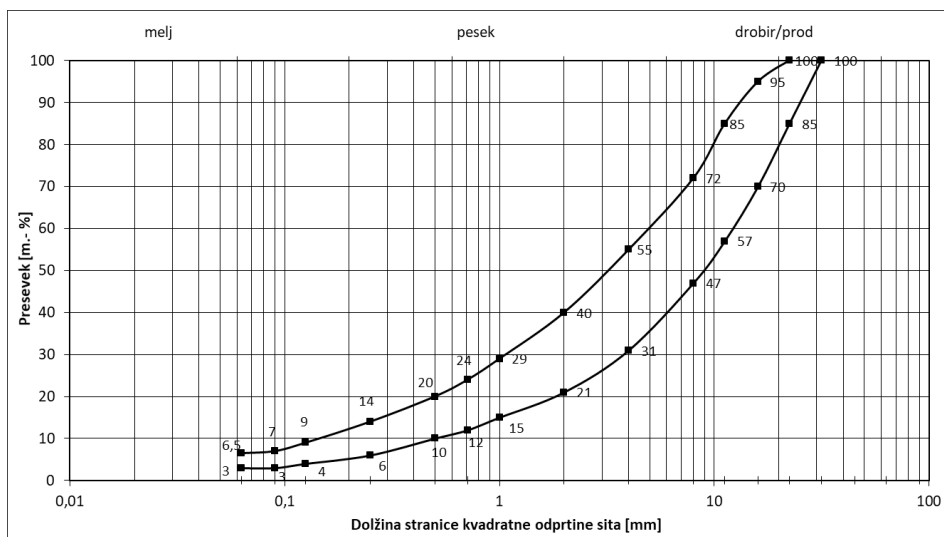
Slika 3.2: Območje sestave agregata 0/22 mm za ZNNP in NOP za vgradnjo
