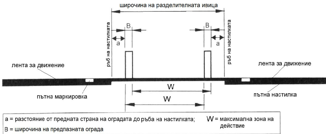
Фигура 17. Едностранны ограничителна система за пътица с разделено действие, разположена до рѐба на настилка
