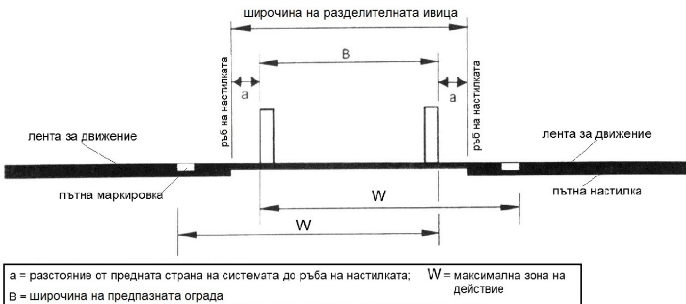
Фигура 18. Едностранны ограничителна система за пътица с общо действие, разположена до рѐба на настилка
