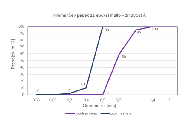
Slika 4.3: Porazdelitev zrnivosti kremenčevega peska A
