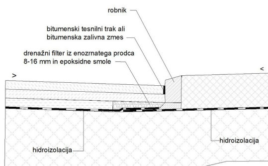
Slika 8.18: Zapolnitev rege ob robnikih in izvedba drenažnega filtra
