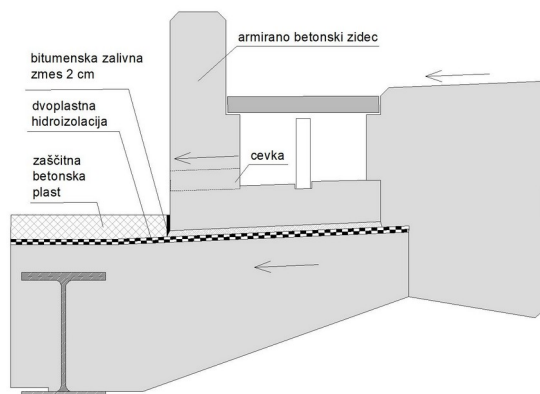
Slika 8.19: Zapolnitev rege ob robnikih na železniških premostitvenih objektih
