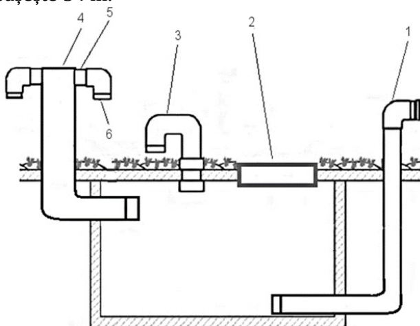
Figura 1. Exemplu de rezervor de apă: 1 – țevă uscată cu manșon de cuplare B(75) de dimensiune PN16 [9.10]; 2 – capac de inspecție care poate fi blocat; 3 – orificiu de ventilație; 4 – tub cu un diametru de 100 mm; 5 – supapă de reținere; 6 – B(75) dimensiune manșon de cuplare PN16 [9.10] pentru realimentarea cu apă.
