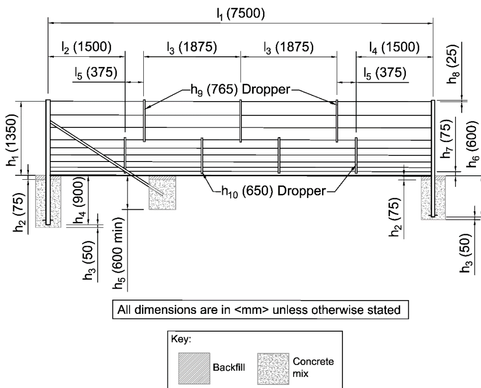
Figure 3.32a Clôture en fil à haute résistance à la traction 1 350
