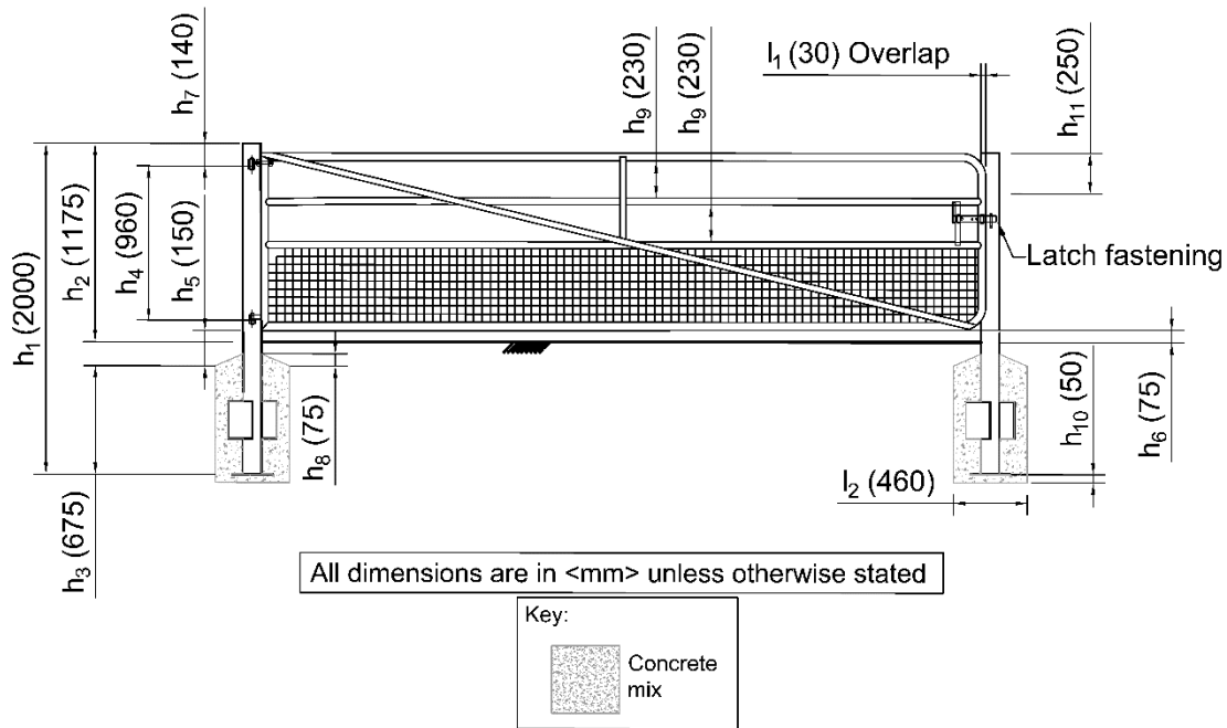
Figure 6.10 sexies Portail de champ en acier doux avec treillis soudé - disposition centrale des charnières
