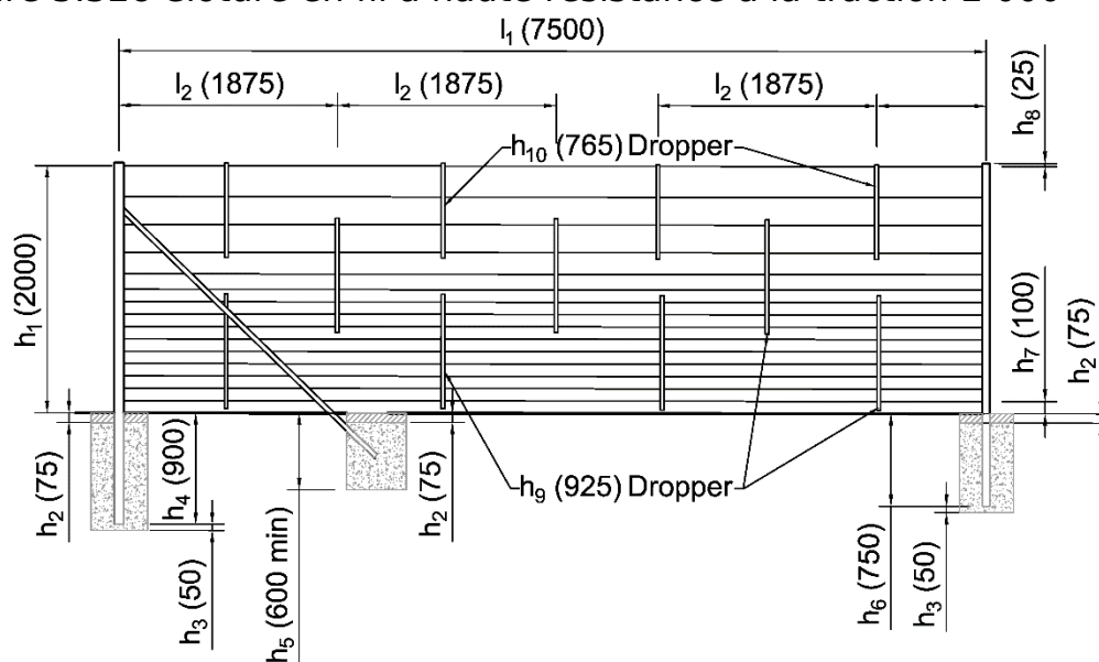
Figure 3.32c Clôture en fil à haute résistance à la traction 2 000
