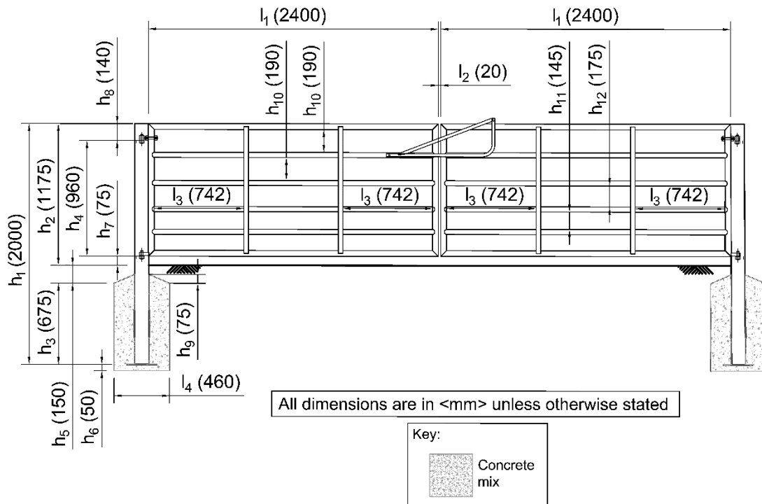
Figure 6.10 septies Portail double de champ en acier doux avec disposition centrale des charnières
