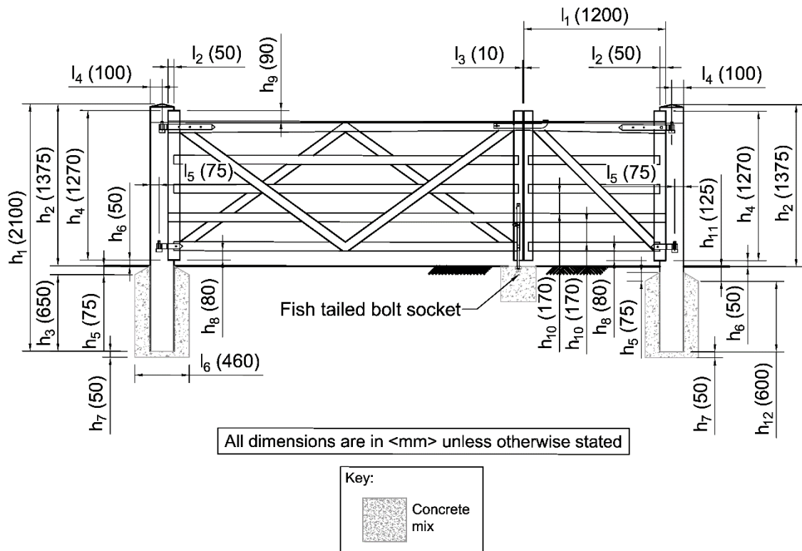
Figure 6.8 ter Portail d'accès au champ en bois et en acier
