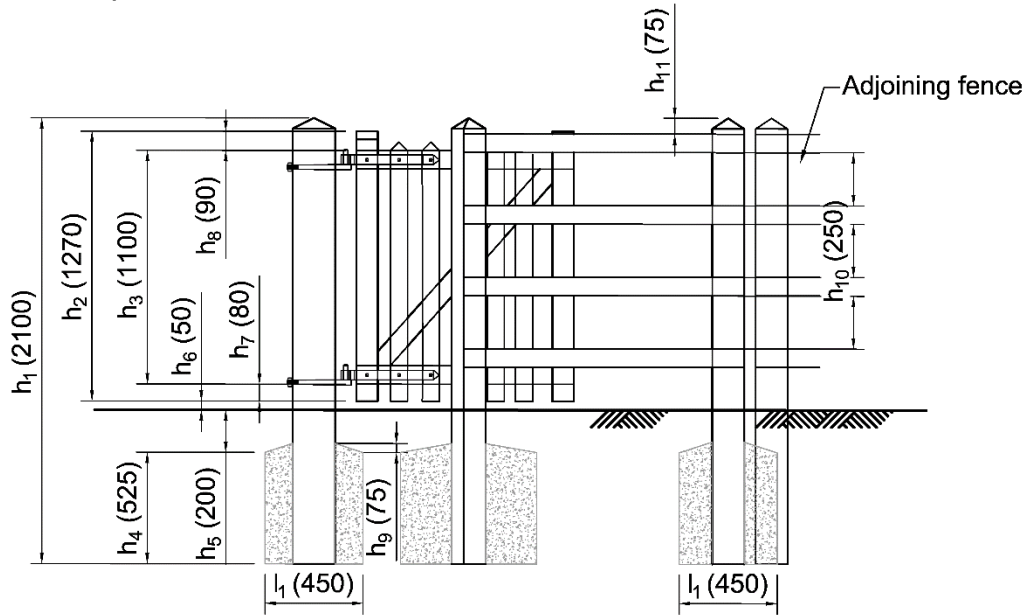
Figure 6.8 quater Portail à embrasser en bois
