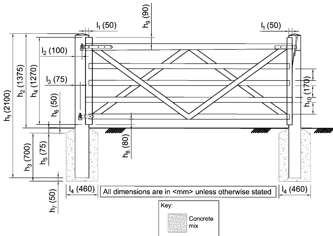
Figure 6.8 bis Portail de champ de bois
