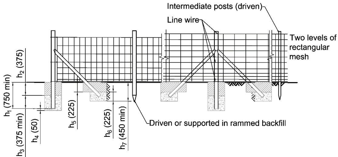
Figure 3.18 Disposition d'installation pour les clôtures en treillis métalliques, treillis hexagonaux en acier et à charnières en fils d'acier tissés
