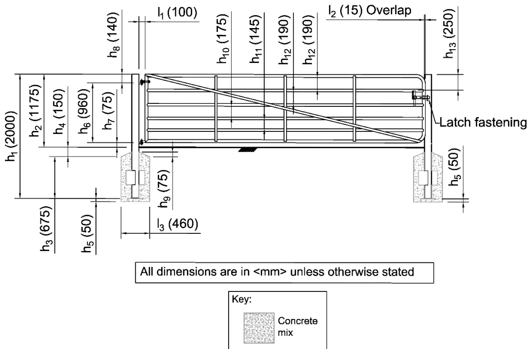
Figure 6.10 bis Portail de champ en acier doux avec disposition latérale des charnières
