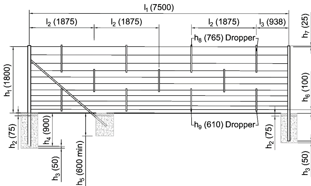
Figure 3.32b Clôture en fil à haute résistance à la traction 1 800
