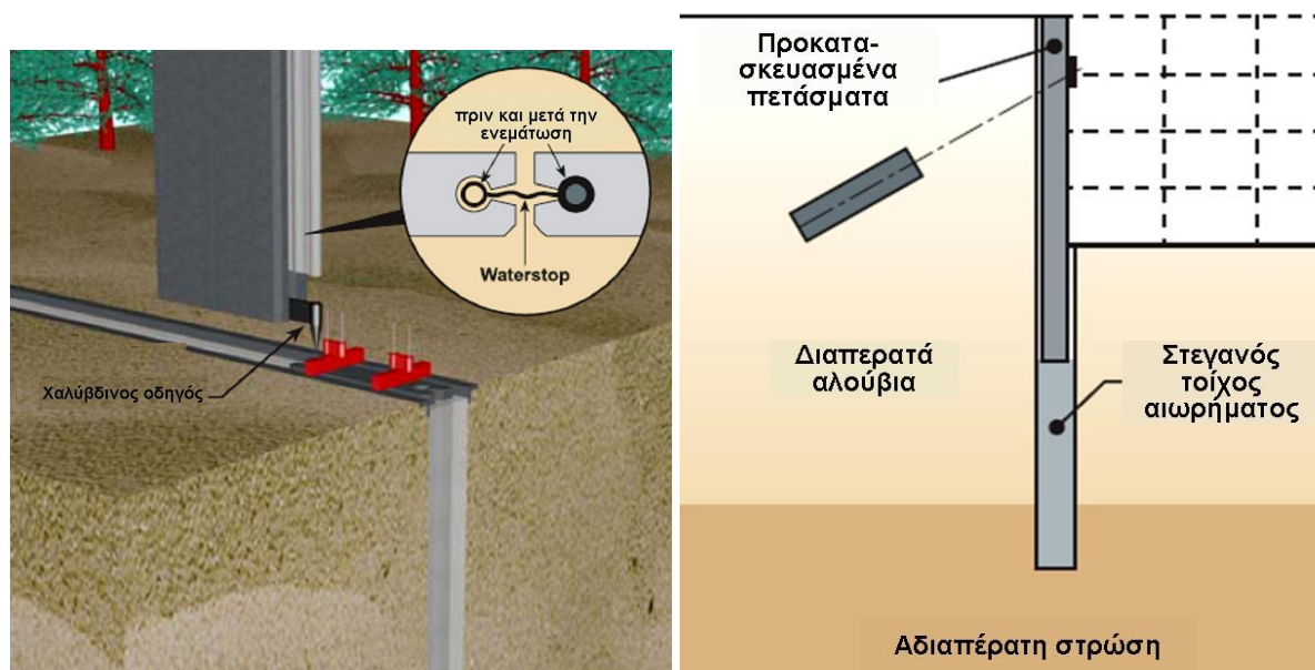
Εικόνα 9 - Διαδικασία κατασκευής πρόχυτων διαφραγματικών τοίχων
