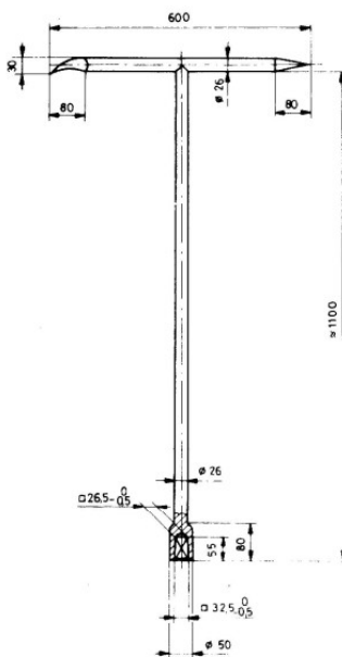
Slika 2. Ključ za nadzemni protupožarni hidrant
