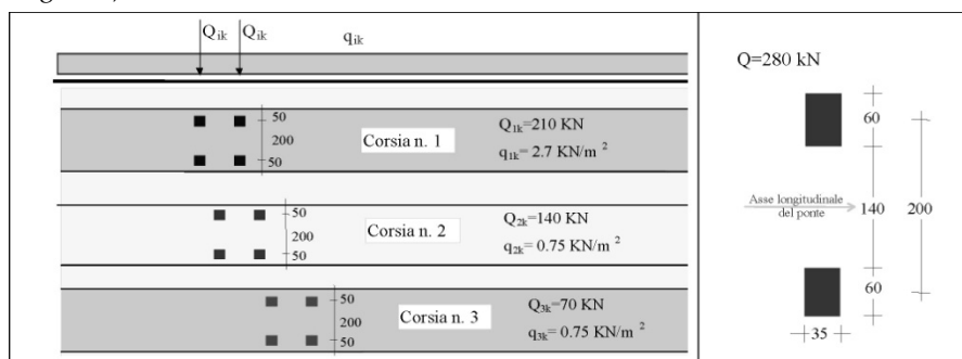
Fig. 5.1.4 - Modello di carico di fatica 1
