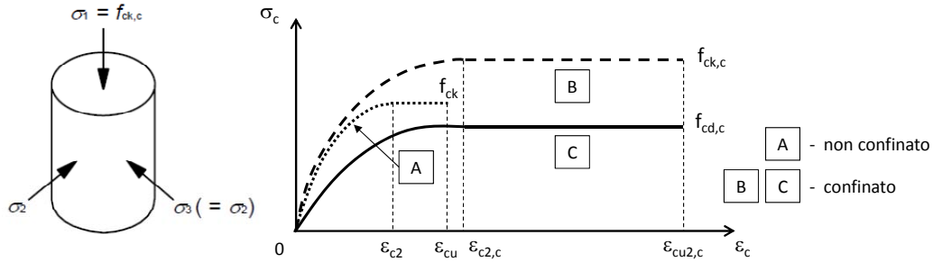
Fig. 4.1.2 – Modelli \sigma - \varepsilon per il calcestruzzo confinato
