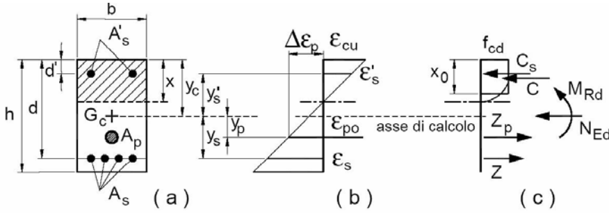
Fig. 4.1.4 – Sezione pressoinflessa
