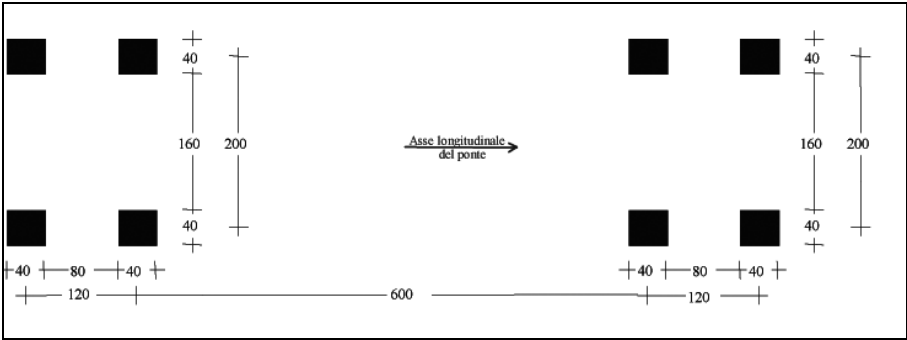
Fig. 5.1.5 - Modello di carico di fatica. 3
