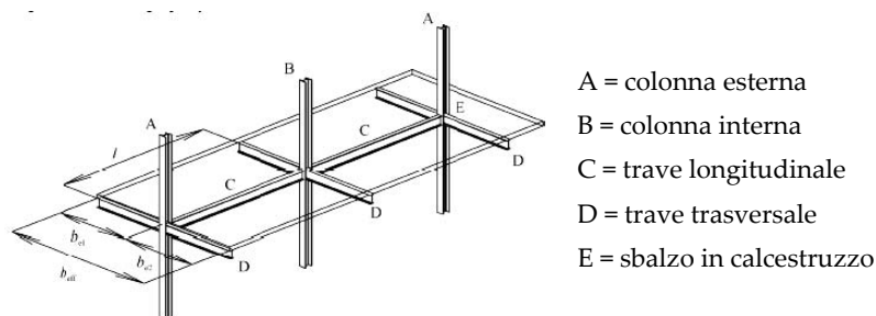
Fig. 7.6.2 - Definizione degli elementi in una struttura intelaiata
