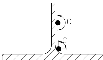
Fig. 4.3.10- Perimetro efficace delle barre di armatura.
