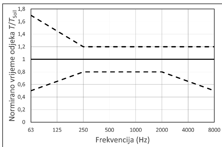
Slika 3 - dopuštena odstupanja od zahtijevanog vremena odjeka T_{\text{Soll}}
