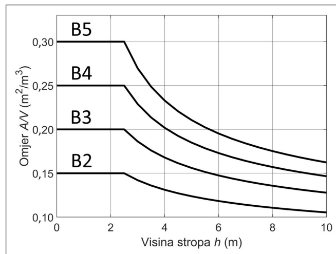
Slika 4 - Minimalne potrebne vrijednosti omjera A/V za pojedine tipove prostoriya kategorije B u ovisnosti o visini stropa h .
