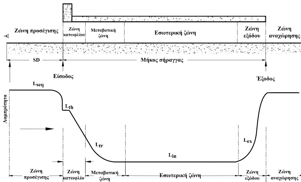
Εικόνα 17: Ζώνες φωτισμού σήραγγας και τυπική διακύμανση λαμπρότητας οδοστρώματος.
