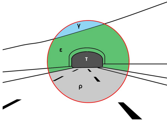
Εικόνα 15: Παράδειγμα σχεδίου σήραγγας από την απόσταση ασφαλούς ακινητοποίησης για τον υπολογισμό της λαμπρότητας L_{20}
