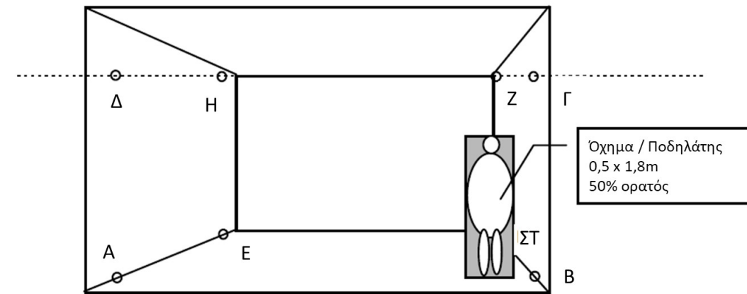
Εικόνα 14: Γενικευμένο σχέδιο εφαρμογής μεθόδου LTP με εμπόδιο πεζό ή ποδηλάτη (παράδειγμα).
