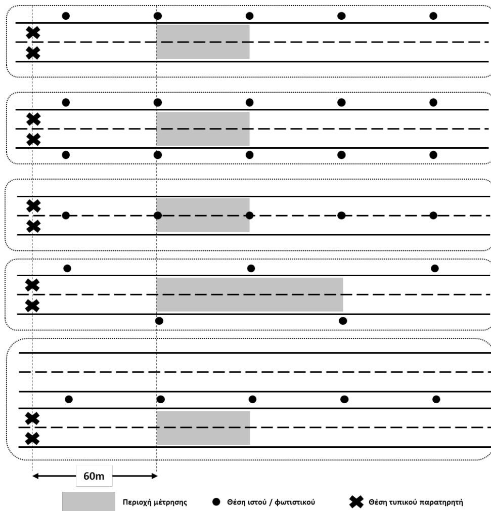
Εικόνα 8 – Τυπικές περιοχές μέτρησης φωτομετρικών χαρακτηριστικών οδοφωτισμού σύμφωνα με το πρότυπο ΕΛΟΤ EN 13201-3 (πηγή TOTEE, 2018).
