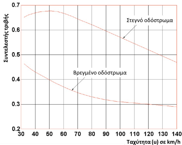
Εικόνα 16: Γραφικός υπολογισμός του συντελεστή τριβής f .
