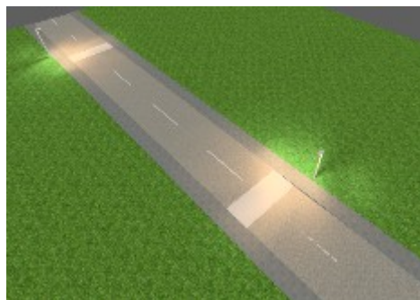
Slika 38: Primer postavitve svetilk za osvetlitev ploščadi trapezne oblike brez prehoda za pešce na neobremenjenem delu ceste znotraj naselja
