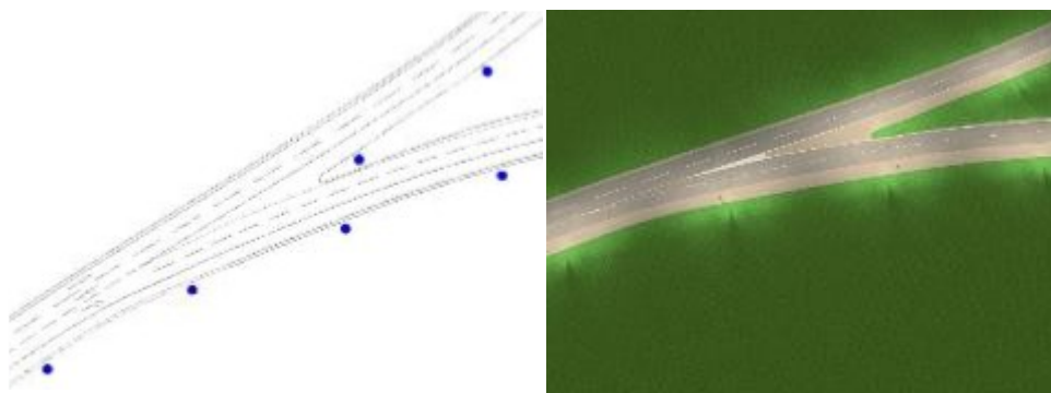
Slika 17: Primer postavitve svetilk za osvetlitev razcepa na avtocesti
