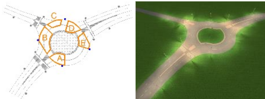
Slika 37: Primer postavitve svetilk za osvetlitev turbo krožnega križišča
