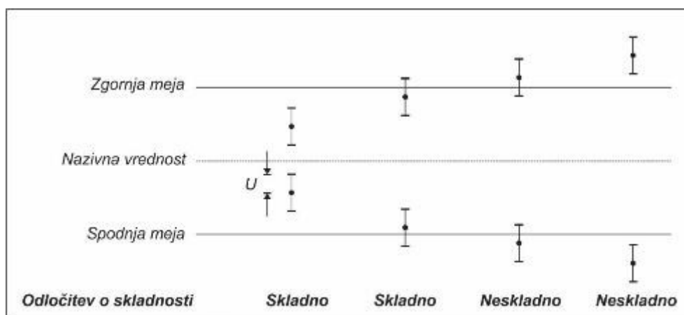
Slika 50: Pravilo odločanja brez upoštevanja merilne negotovosti meritve
