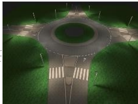
Slika 35: Primer postavitve svetilk za osvetlitev krožnega križišča s samostojnimi prehodi za pešce
