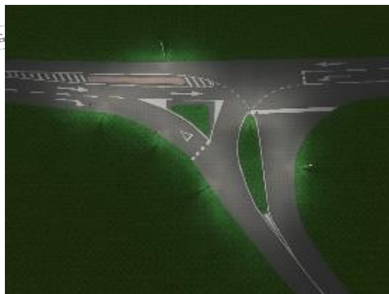
Slika 41: Primer postavitve svetilk za osvetlitev deniveliranih otokov v križišču
