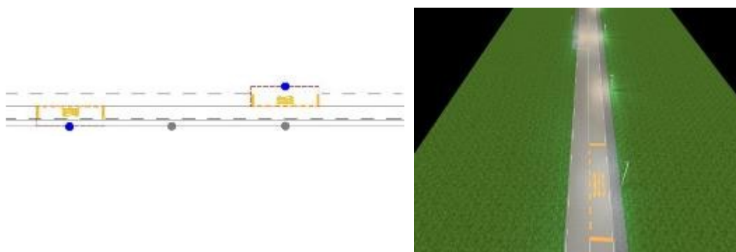
Slika 25: Primer postavitve svetilk za osvetlitev avtobusnih postajališč na neobremenjenem delu ceste z eno svetilko
