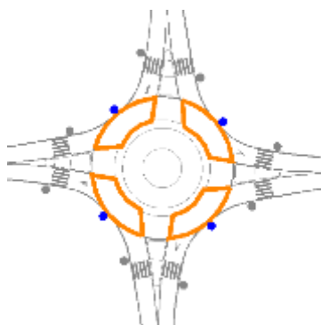
Slika 35: Primer postavitve svetilk za osvetlitev krožnega križišča s samostojnimi prehodi za pešce
