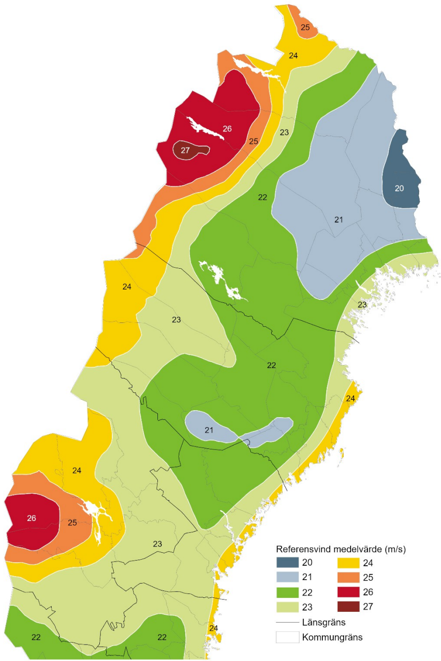
Figur 4:3. Referensvindhastighet, v_b
